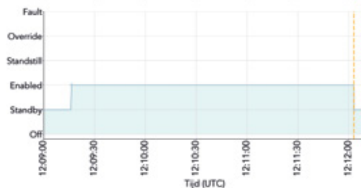
Figuur 26: Tijdreeksregistratie van een aantal parameters afkomstig van de logbestanden uit het voertuig (Tesla Model S, Ouddorp).
