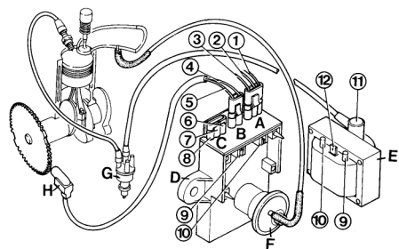
Figuur 8.1: Overzicht elektronisch ontstekingsysteem
